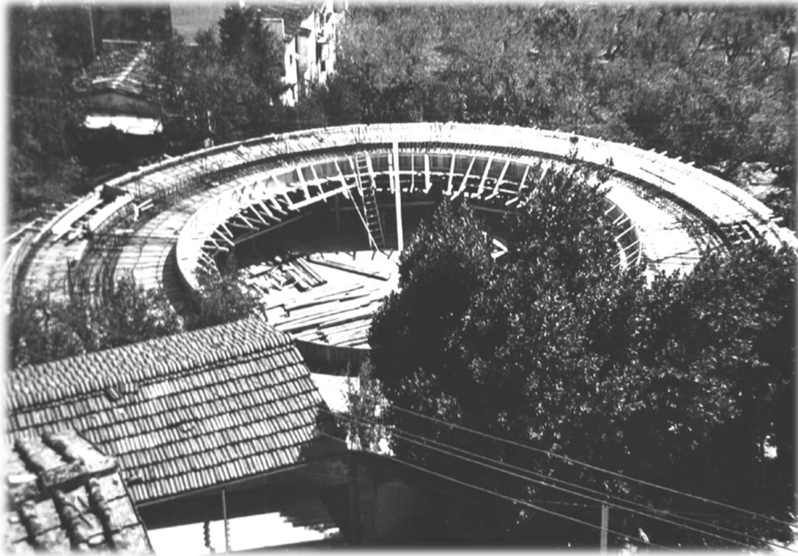
Settignano 1960 : costruzione del tetto della Rotonda
